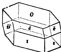
Miask, Ural.
